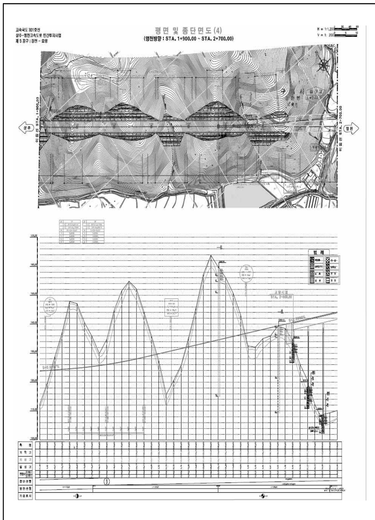
【그림 30.3】 평면도
