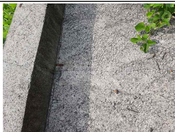
소단배수로 균열
