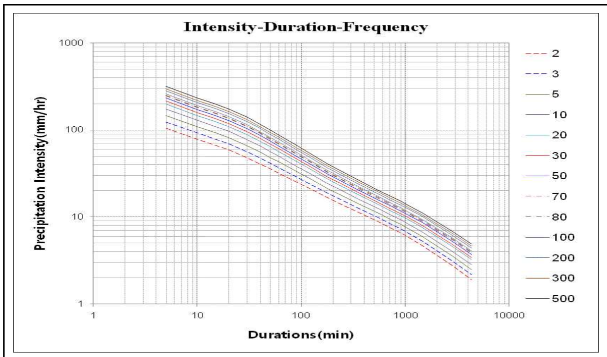
【그림 30.9】 균위지역 IDF곡선
