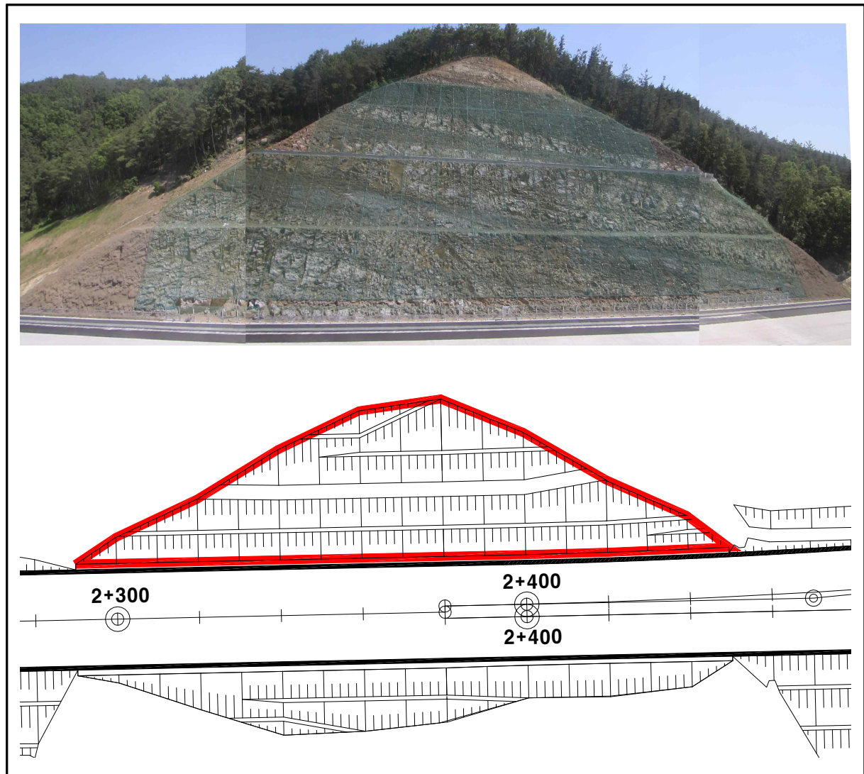
【그림 30.14】 상주절토30 검토대상 비탈면구간
